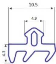
AP 03 3MM E TYPE
